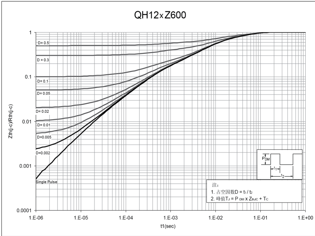
图10. 归一化最大动态热阻抗
