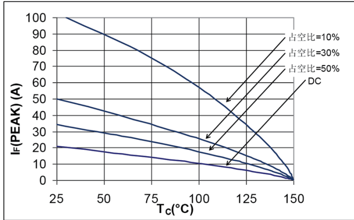
图9. I_F (峰值)相对于 T_c 的变化, f = 70\text{kHz}
