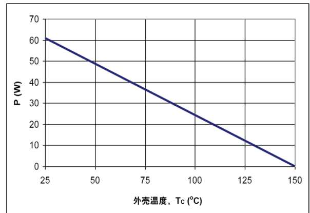
图8. 功率降额曲线
