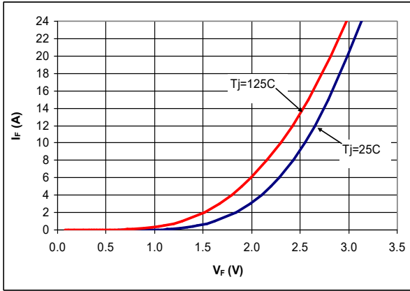
图3. I_F 相对于 V_F 的典型变化
