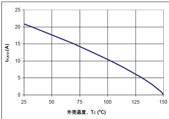
图7. 直流电流降额曲线
