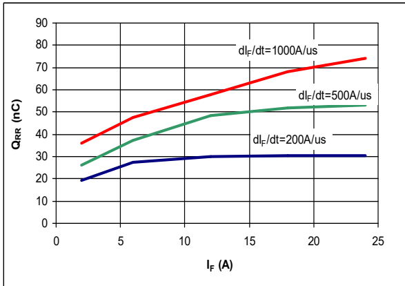
图5. Q_{RR} 相对于 I_F 的典型变化, T_J = 125^\circ\text{C}
