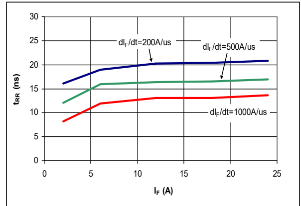
图6. t_{RR} 相对于 I_F 的典型变化, T_J = 125^\circ\text{C}
