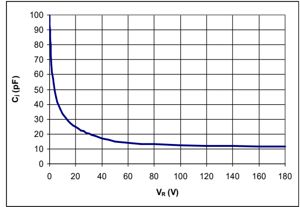
图4. C_J 相对于 V_R 的典型变化
